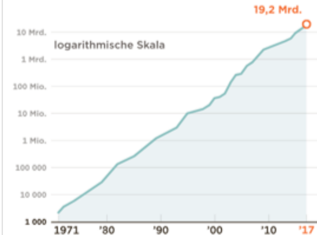
Zahl der Transistoren, die in einen Mikroprozessor passen
